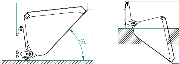
Grand angle de basculement pour un remplissage et une vidange parfaits
