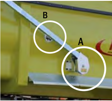
Entraînement hydraulique via moteur hydraulique – pour rentrer le filet
