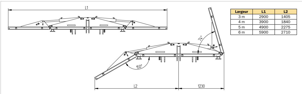
Largeur de déblayage réglable en continu par les 2 panneaux latéraux, grillage de rehausse (en option)
