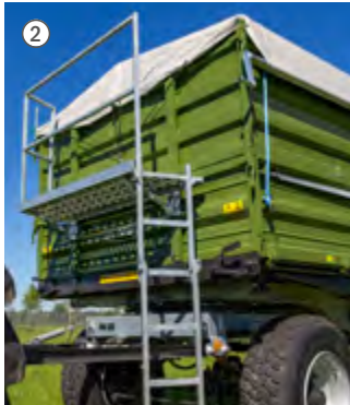
Avec échelle dépliable
