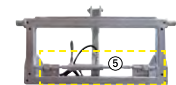
③ + ④ Adaptateur trois points, à verrouillage hydraulique
