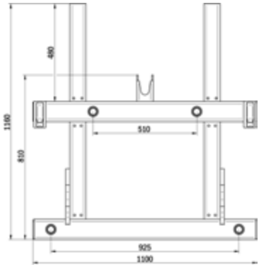
Version avec rehausse et 4 dents de balle ronde (2 dents de série)
